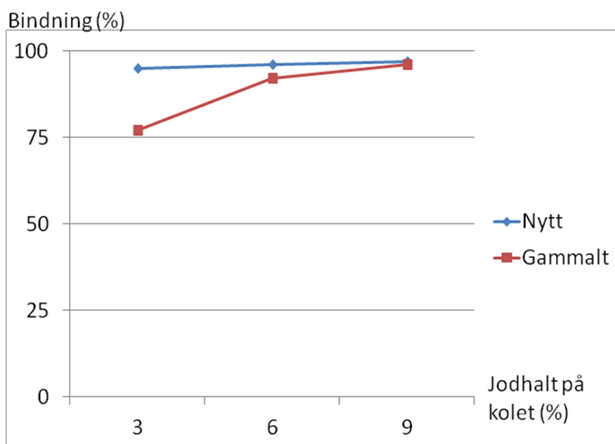
Fig 2: Kviksilverbindning för ny och gammal typ av Iodocarb.
